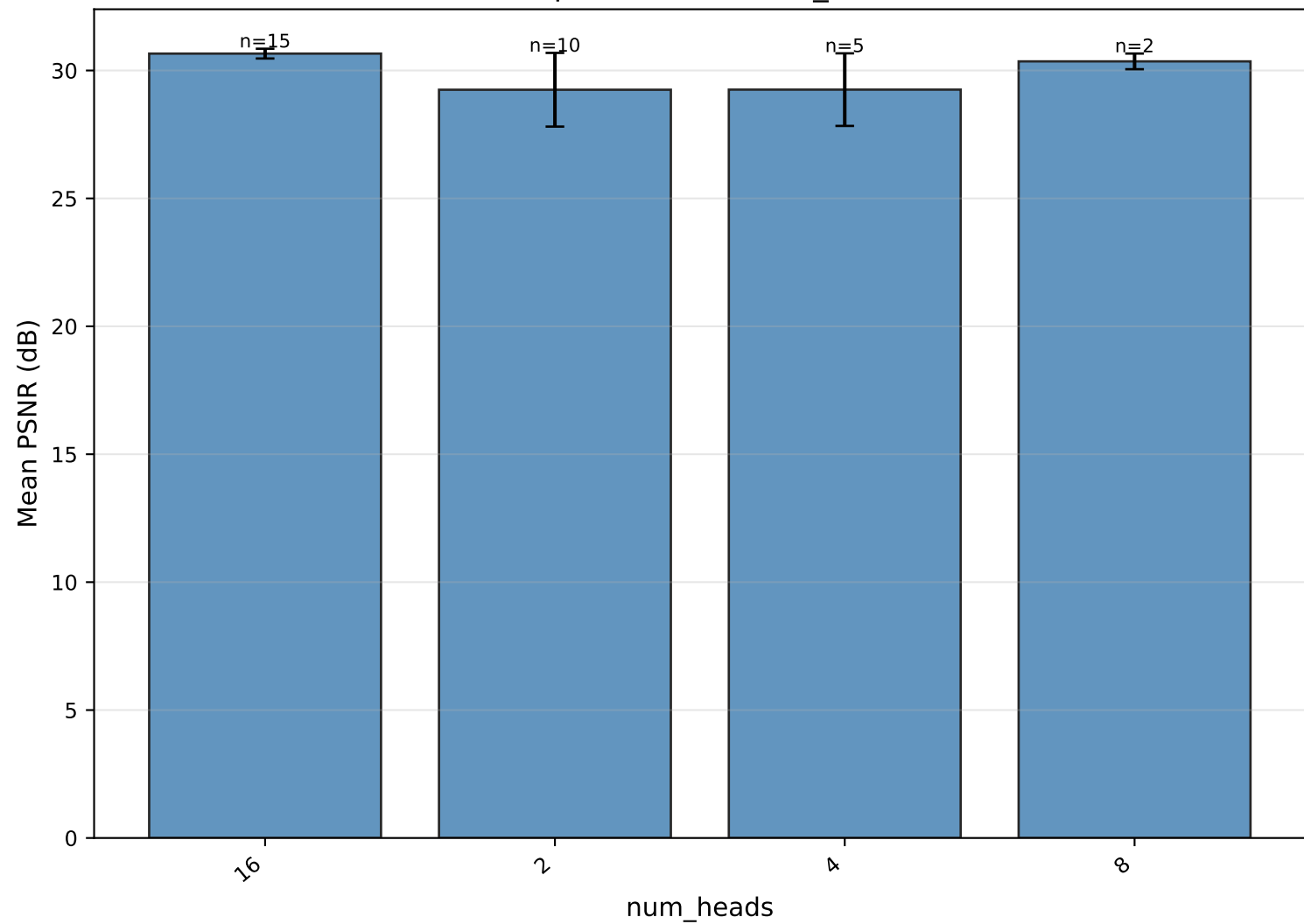
Mean PSNR per value of num_heads — DAT
